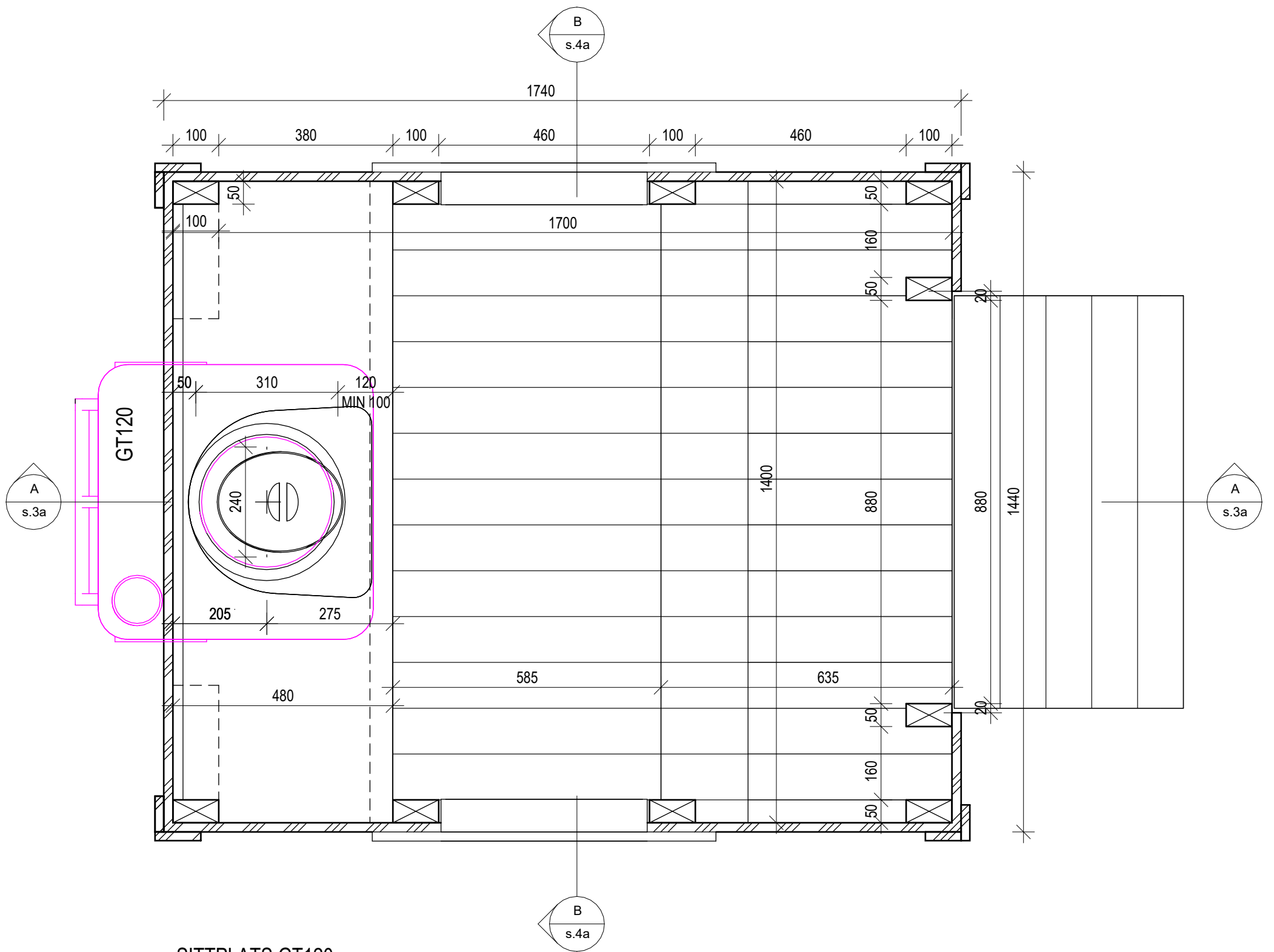
SITTPLATS GT120
