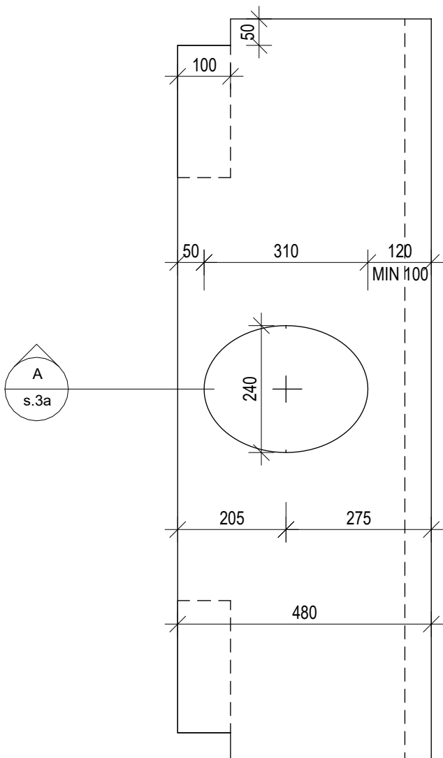
SITTPLATS GT120
