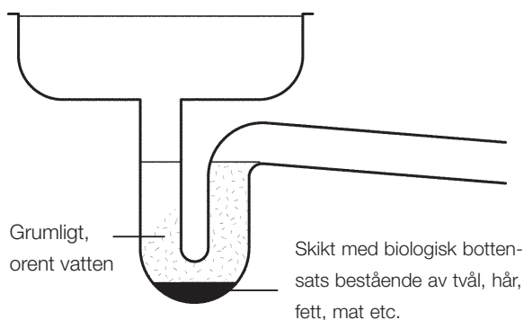
Figur 1. Nackdelen med stillastående vatten i ett traditionellt vattenlås
